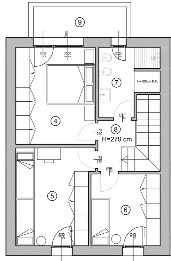
PIANO PRIMO
